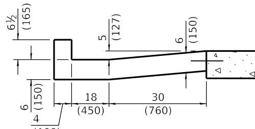
SECTION D-D
