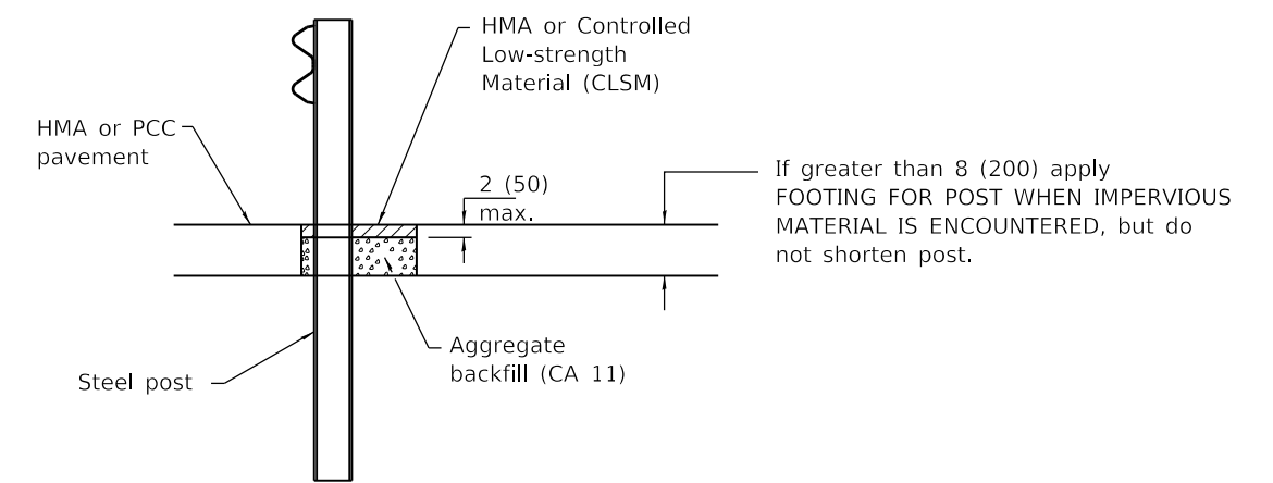
ELEVATION
