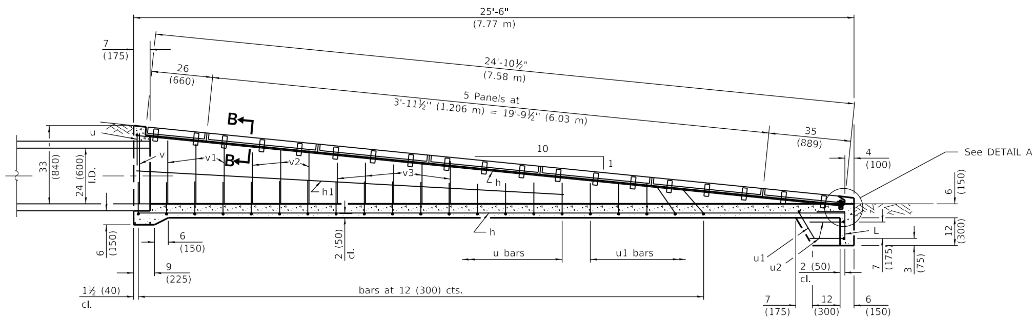
SECTION A-A
