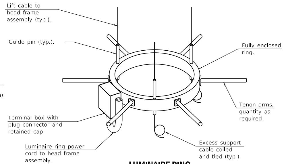
LUMINAIRE RING
