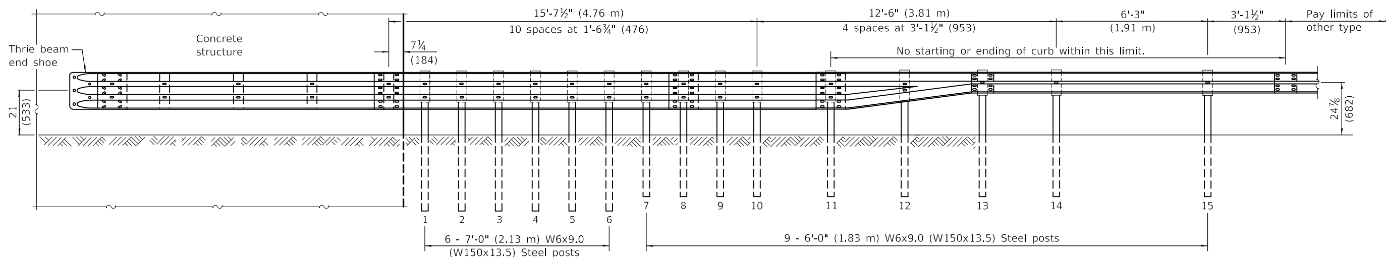
ELEVATION
