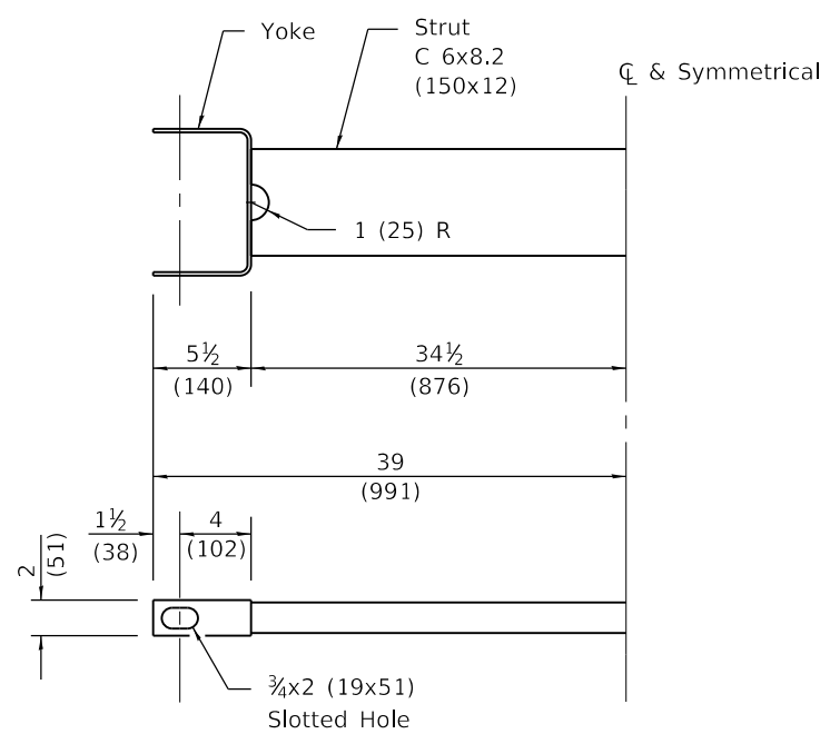
CABLE STRUT
