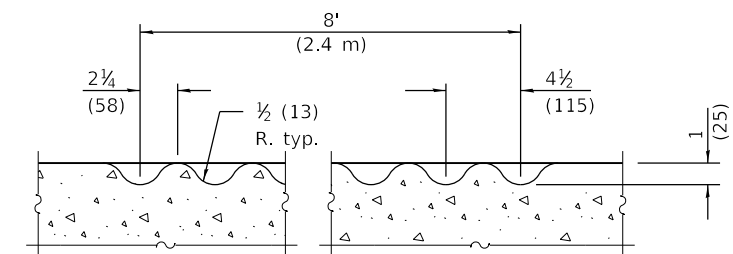
SECTION D-D
