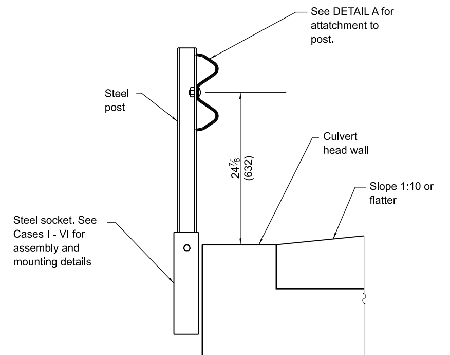
SECTION A-A
