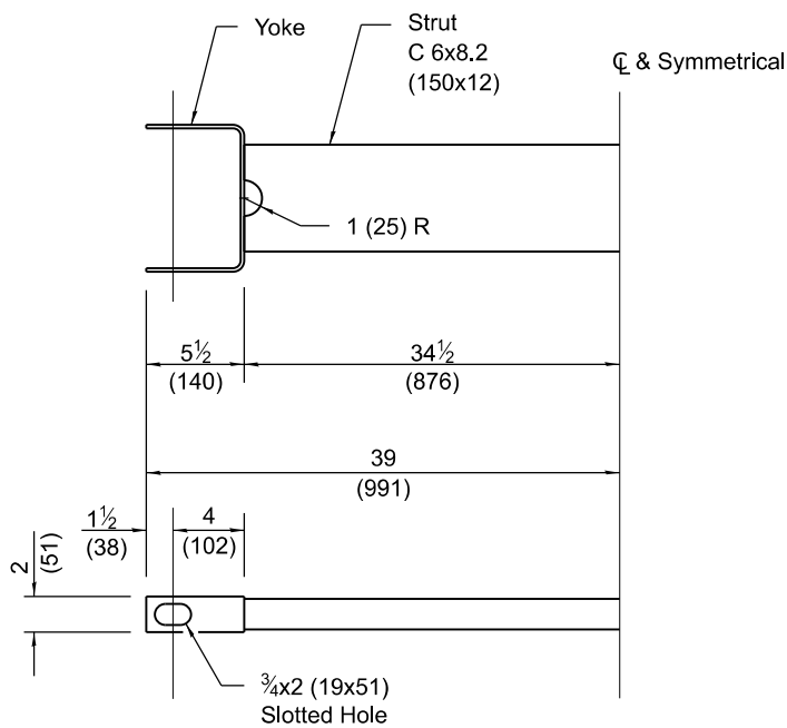
CABLE STRUT
