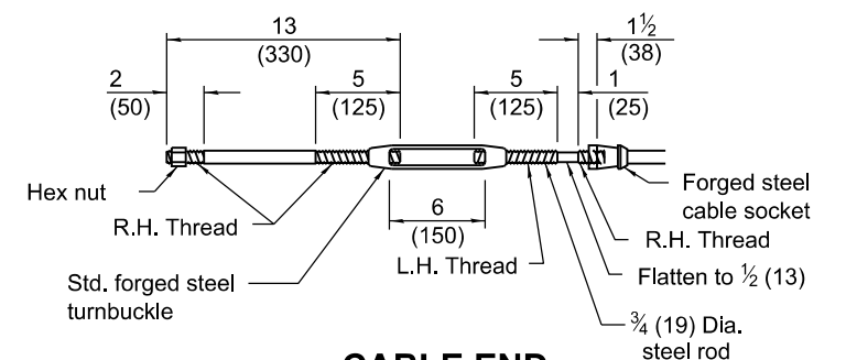
CABLE END
