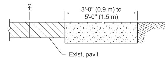
SECTION D-D
